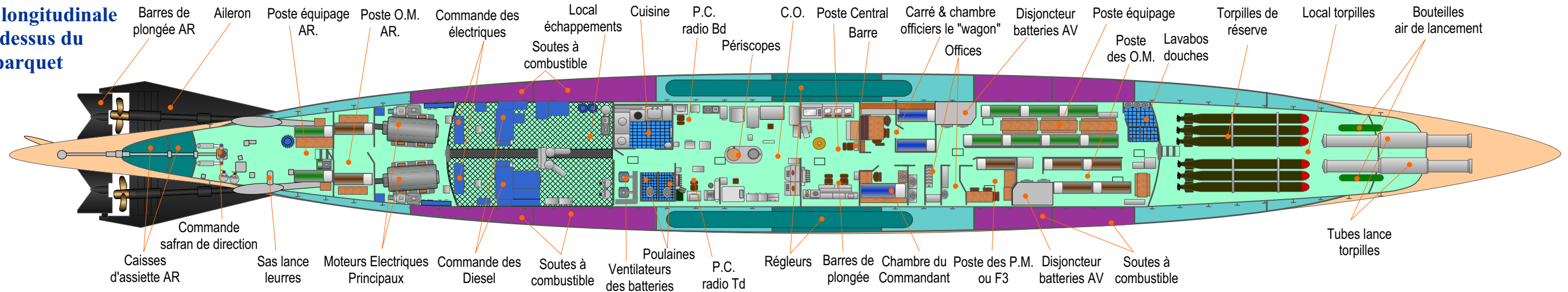
Coupe longitudinale au dessous du parquet
